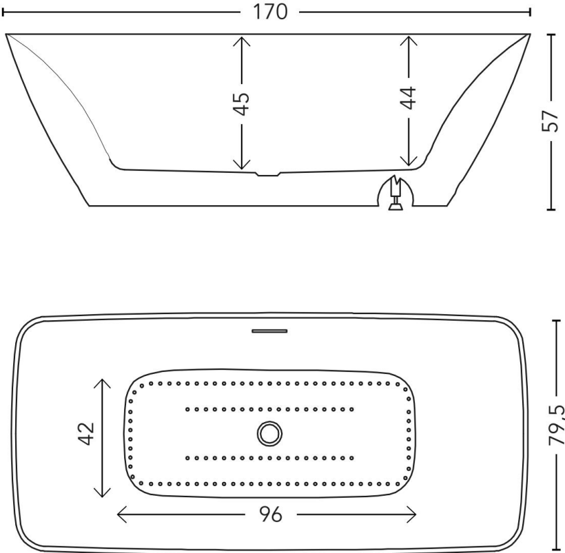
medidas: cm
