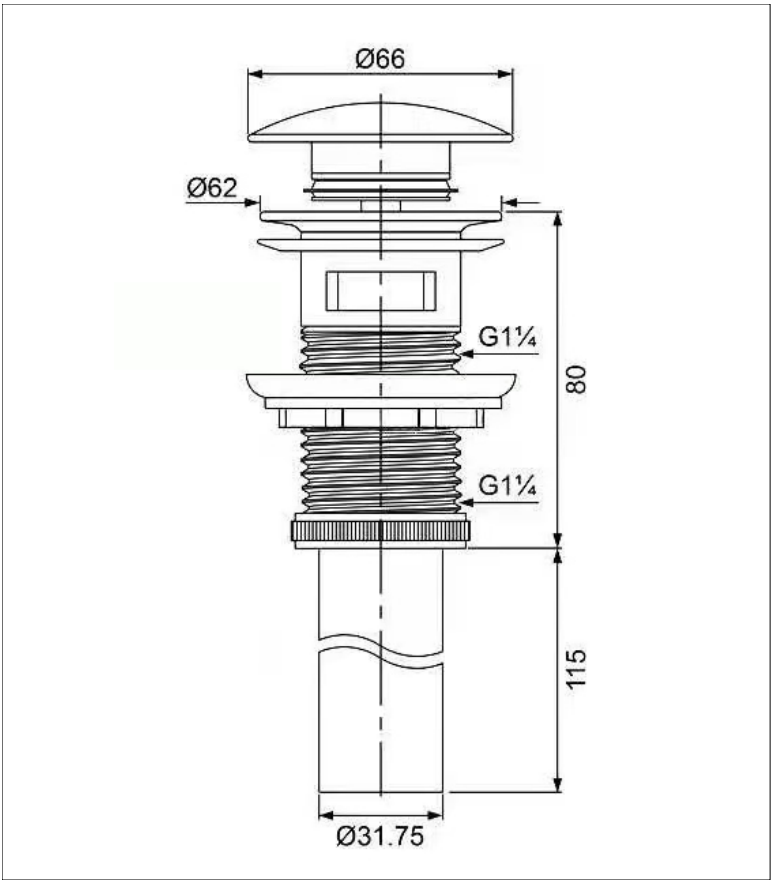
Válvula click
