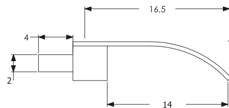
Cascata - vista lateral
