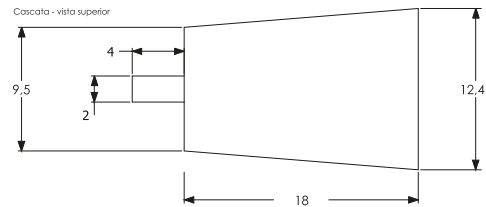
Cascata - vista superior
