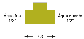
Corpo do monocomando - vista superior
